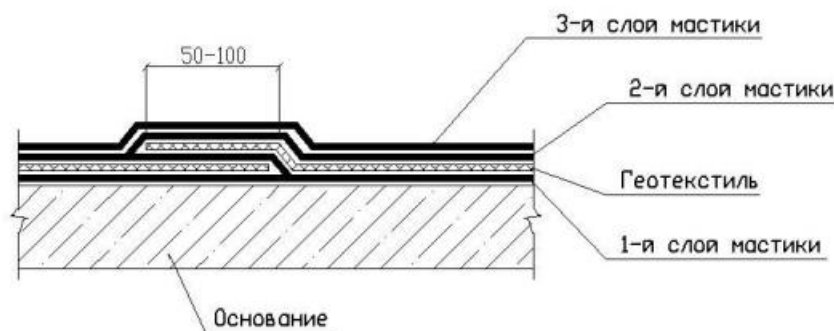
Рисунок 7 – Укладка полотен геотекстиля с нахлестом
