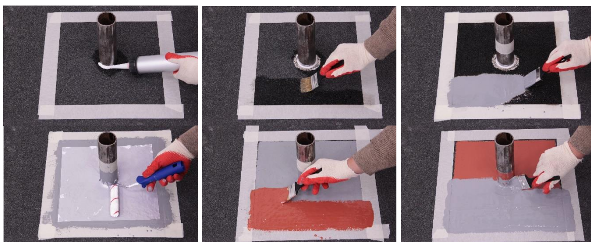
Рисунок 8 – Примыкание водоизоляционного слоя покрытия к холодным трубам из материалов, к которым у мастики имеется адгезия
