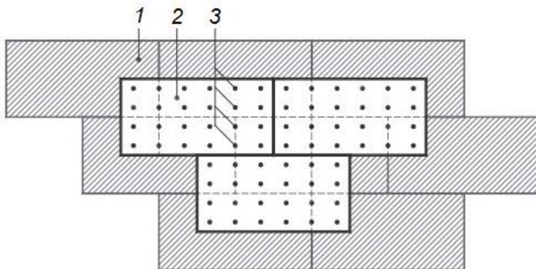
Рисунок 6 – Схема крепления листов сборной стяжки из ХЦЛ (ЦСП)
