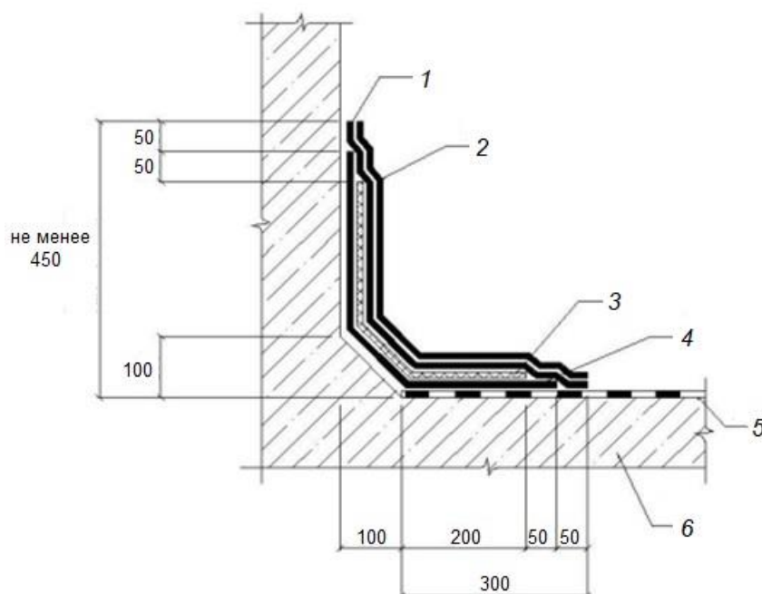
Рисунок 14 – Выполнение примыкания битумной мастикой после нанесения основного водоизоляционного слоя с одним слоем геотекстиля
