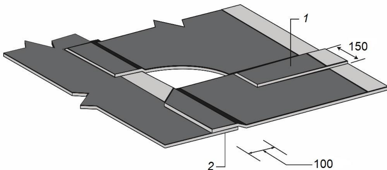
1 – поперечный шов; 2 – продольный шов
