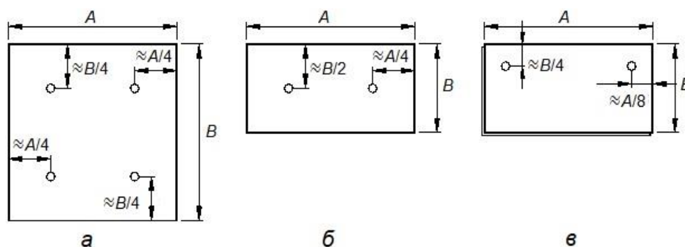
Рисунок 3 – Схема крепления теплоизоляционных плит
