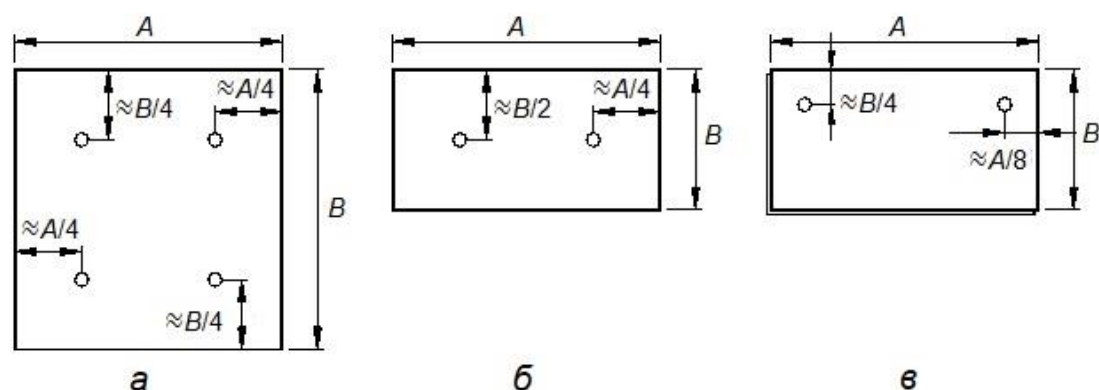
Рисунок 4 – Схема крепления теплоизоляционных плит:
