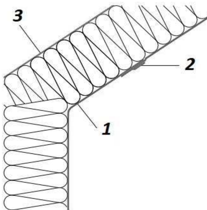
1 – пароизоляционная пленка; 2 – соединительная лента; 3 – диффузионная пленка Рисунок 2 – Схема укладки пароизоляционной пленки поперек стропильных ног
