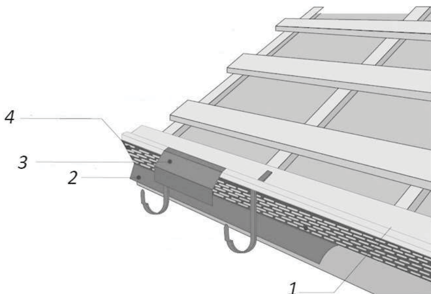
1 – первая доска обрешетки; 2 – капельник; 3 – карнизная планка; 4 – вентиляционная сетка
