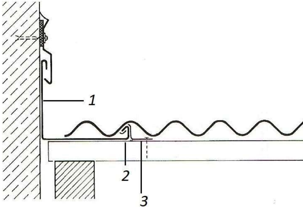
Рисунок 15 – Пример крепления планки примыкания нижней
