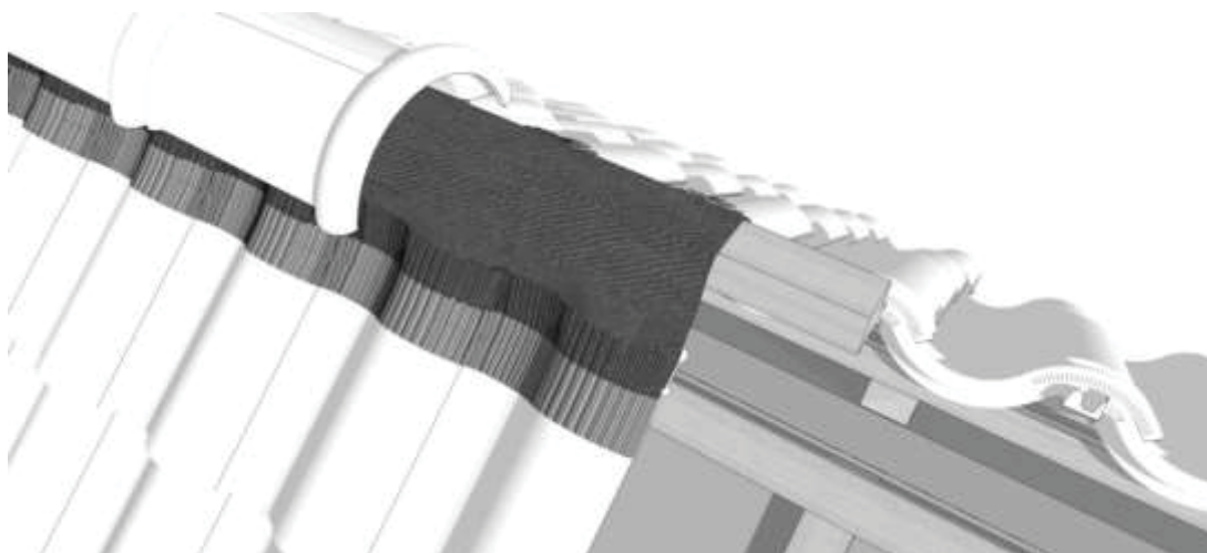
Рисунок 13 – Пример установки рулонного аэроэлемента конька
