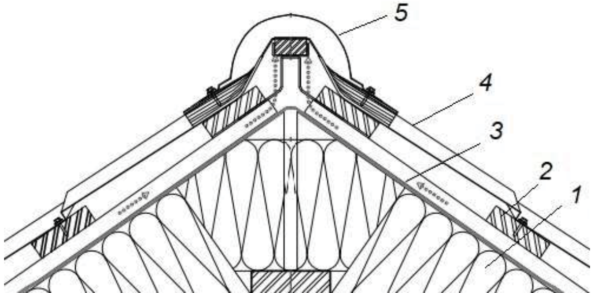
1 – теплоизоляционные минераловатные плиты (маты); 2 – контробрешетка; 3 – диффузионная пленка; 4 – металлочерепица; 5 – коньковый элемент Рисунок 5 – Укладка диффузионной пленки на коньке утепленной крыши с одним вентиляционным зазором
