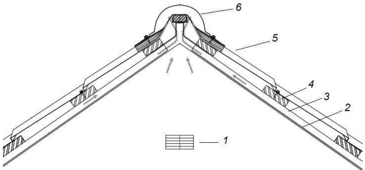
1 – слуховое окно или продух; 2 – водозащитная пленка; 3 – обрешетка; 4 – контробрешетка; 5 – металлочерепица; 6 – коньковый элемент Рисунок 6 – Укладка водозащитной пленки на коньке холодной крыши с утеплением по чердачному перекрытию
