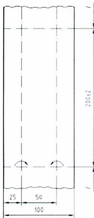
Рисунок В.1 – Складывание образца для испытаний
